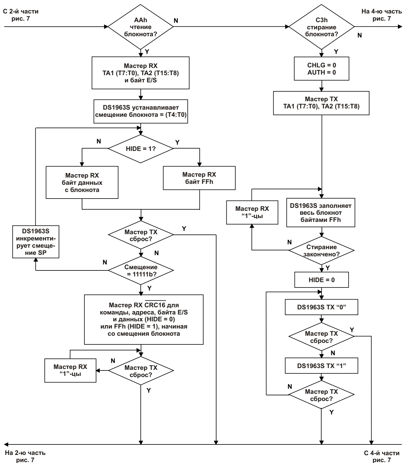
Рис. 7-3. БЛОК-СХЕМА ФУНКЦИЙ ПАМЯТИ И SHA (продолжение)
