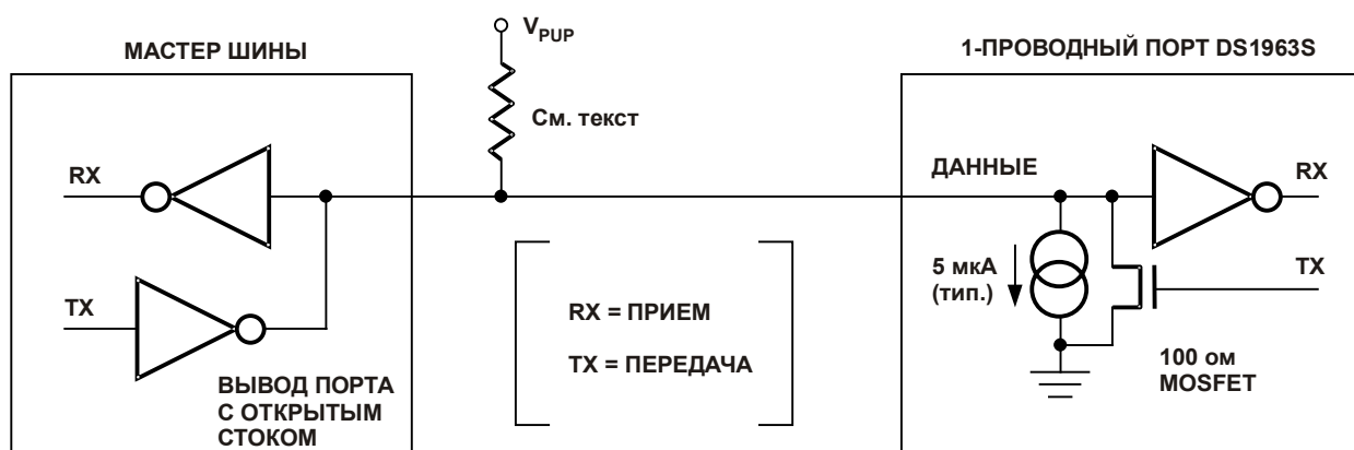
Рис. 9. АППАРАТНАЯ КОНФИГУРАЦИЯ
