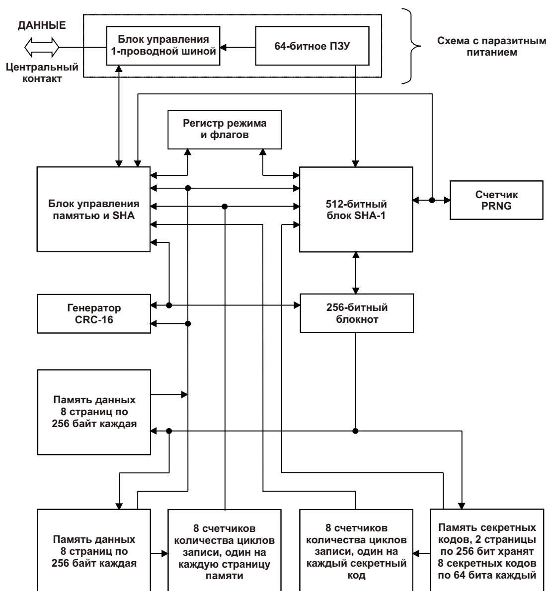
Рис. 1. БЛОК-СХЕМА DS1963S
